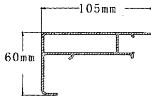
Seitenrahmen Seitenansicht
